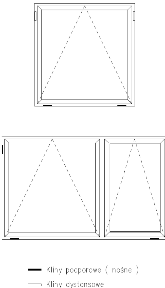
Rys. 12 Rozmieszczenie minimalnej liczby klinów podporowych i dystansowych.
