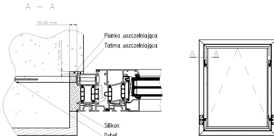
Rys. 8 Okno w ścianie z węgarkiem zewnętrznym.
