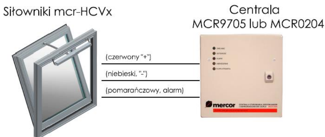
Rys. 14 Schemat połączeniowy siłowników mcr-HCVx.
