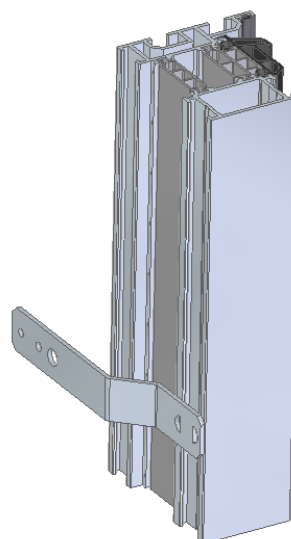
Rys. 7 Montaż za pośrednictwem kotew.
