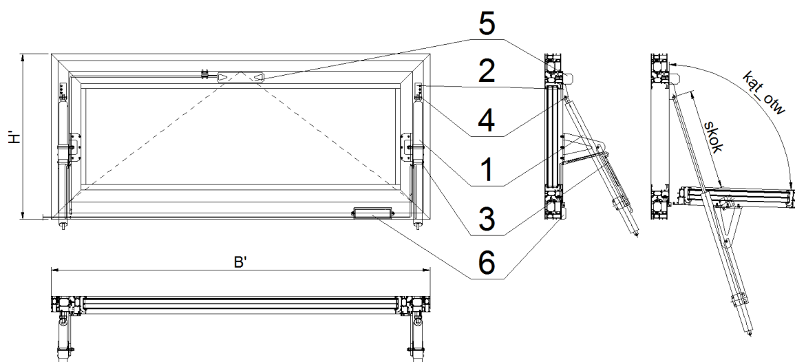
1 – siłowniki wrzecionowe, 2 – uchwyt górny, 3 – uchwyt dolny z zaczepem i obejmą przesunięcia punktu obrotu, 4 – trzpień górny, 5 – elektorygiel obrotowy, 6 – interfejs rygla
